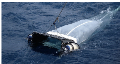
ニューストンネットを用いたマイクロプラスチックの採集 Floating microplastic sampling using a neuston net
