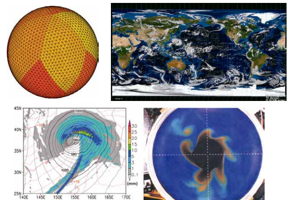
全球非静力学モデルNICAMの開発 (左上)と数値実験で得られた全球の雲分布 (右上)。数値シミュレーションで再現された爆弾低気圧 (左下)と回転系の水平対流の室内実験 (右下)。 Global nonhydrostatic model, NICAM (upper left), global cloud distribution simulated by NICAM (upper right), numerically simulated explosively-developing extratropical cyclone (lower left), and horizontal convection in a rotating tank experiment (lower right)
