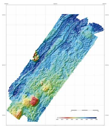
自航式深海探査機でとらえたマリアナ背弧海底拡大軸の詳細地形
