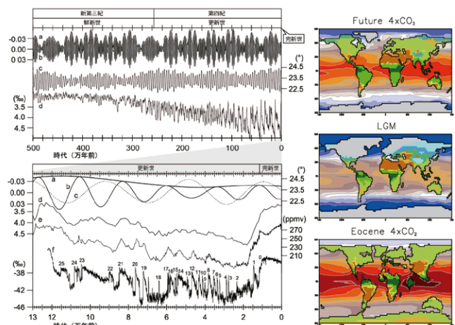
過去500万年の気候変化(左)と気候モデルMIROCによる気候シミュレーション(海面水温と植生分布)例(右、将来CO 2 4倍想定(上)、2万年前の最終氷期(中)、5500万年CO 2 4倍の場合(下))。
