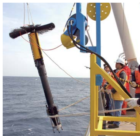
白鳳丸における乱流計回収作業風景
