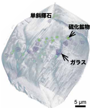
図4 鉱物中に含まれる極微小包有物の3D解析結果 Fig. 4 3D investigation of sub- \mu m-sized inclusion array
