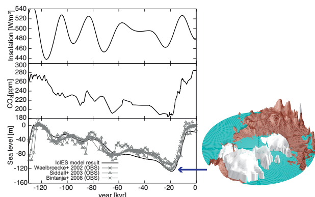
過去約12万年前からの最終氷期サイクルにおける、日射、二酸化炭素濃度、海水準の変化 (OBS: 観測, lclES: シミュレーション) とモデルにより再現された最終氷期最盛期の氷床の鳥瞰図
