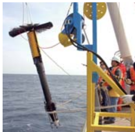
白鳳丸における乱流計回収作業風景
